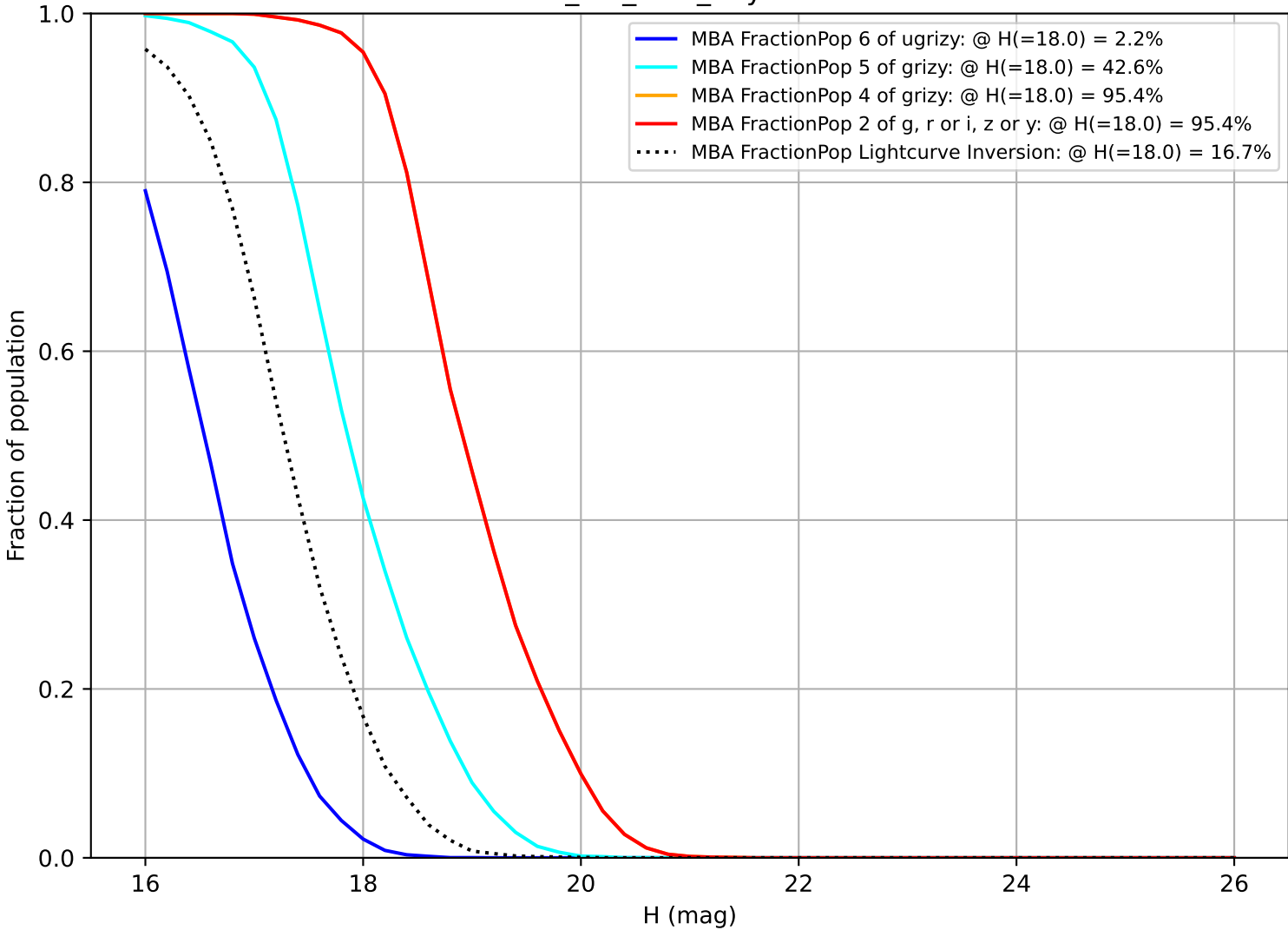
ddf_roll_v3.5_10yrs MBA
