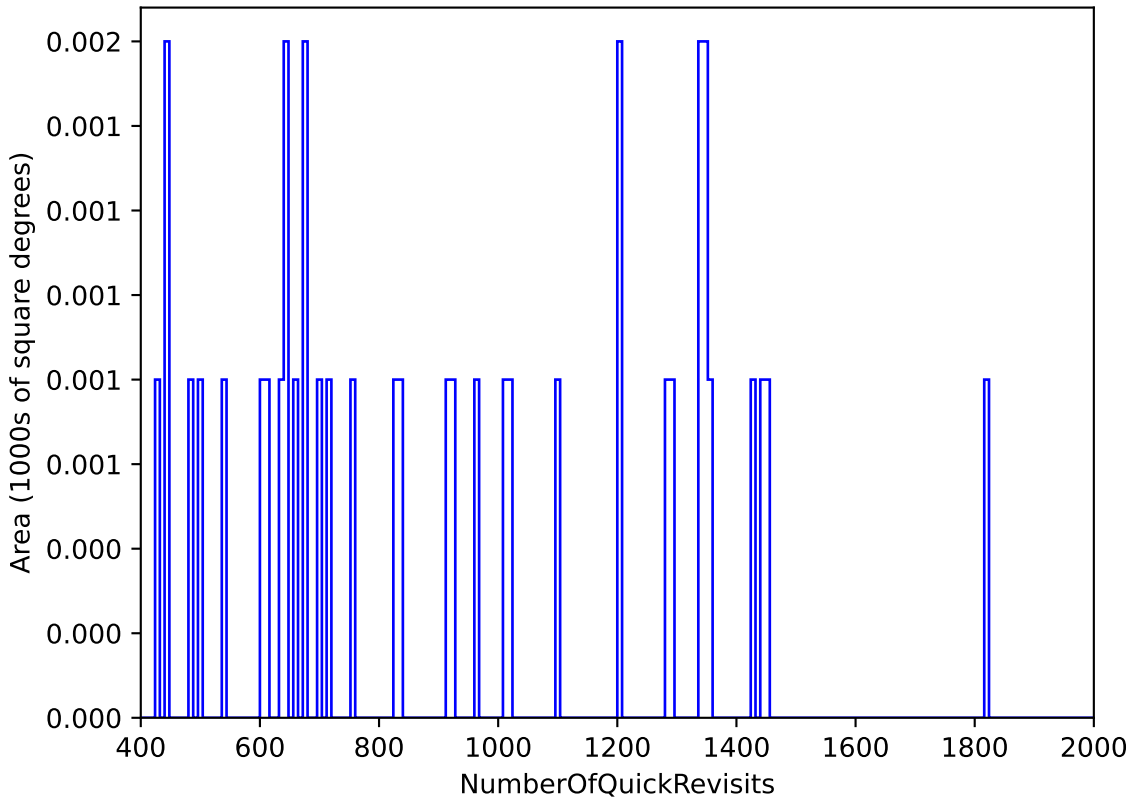
four_cycle_v3.5_10yrs : NumberOfQuickRevisits
