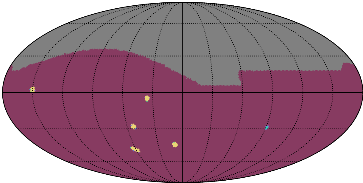
four_cycle_v3.5_10yrs : NumberOfQuickRevisits
