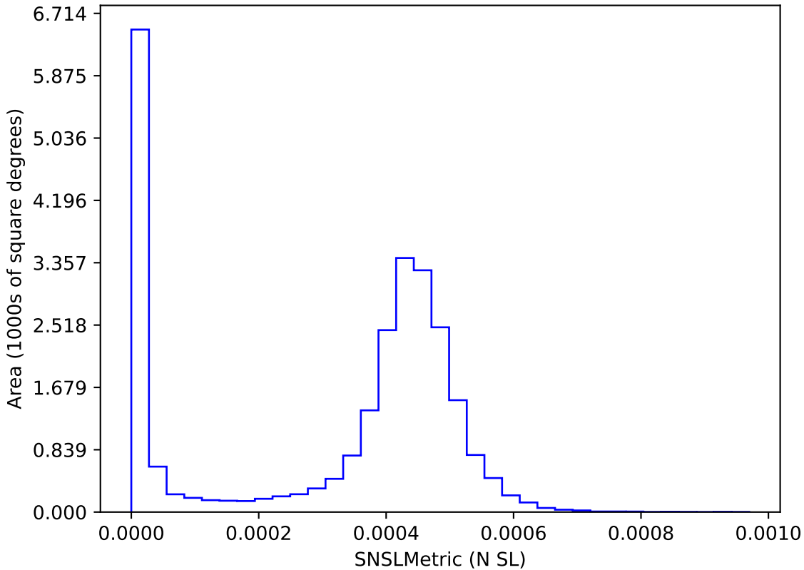
four_cycle_v3.5_10yrs : SNSLMetric
