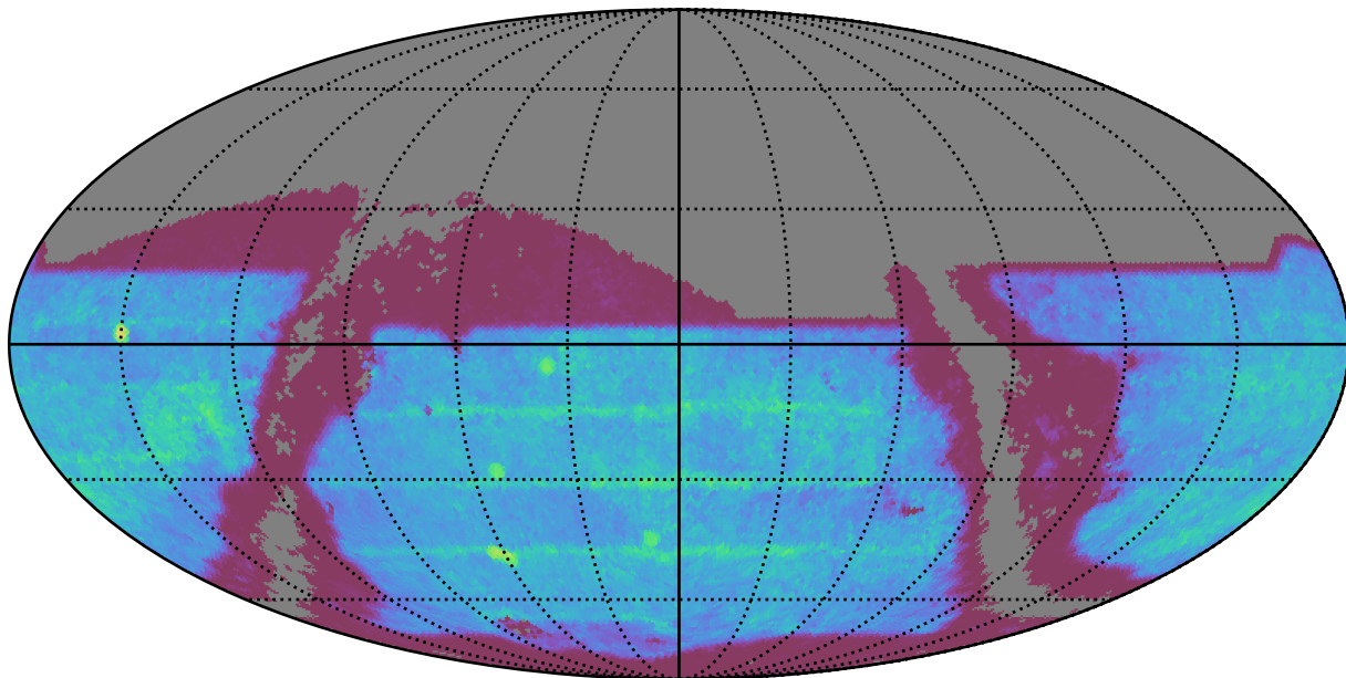
four_cycle_v3.5_10yrs : SNSLMetric
