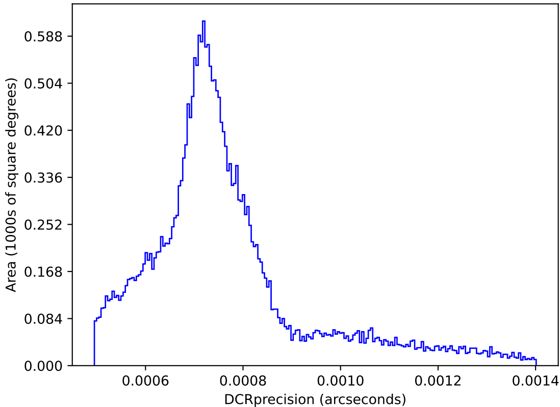
four_cycle_v3.6_10yrs : DCRprecision
