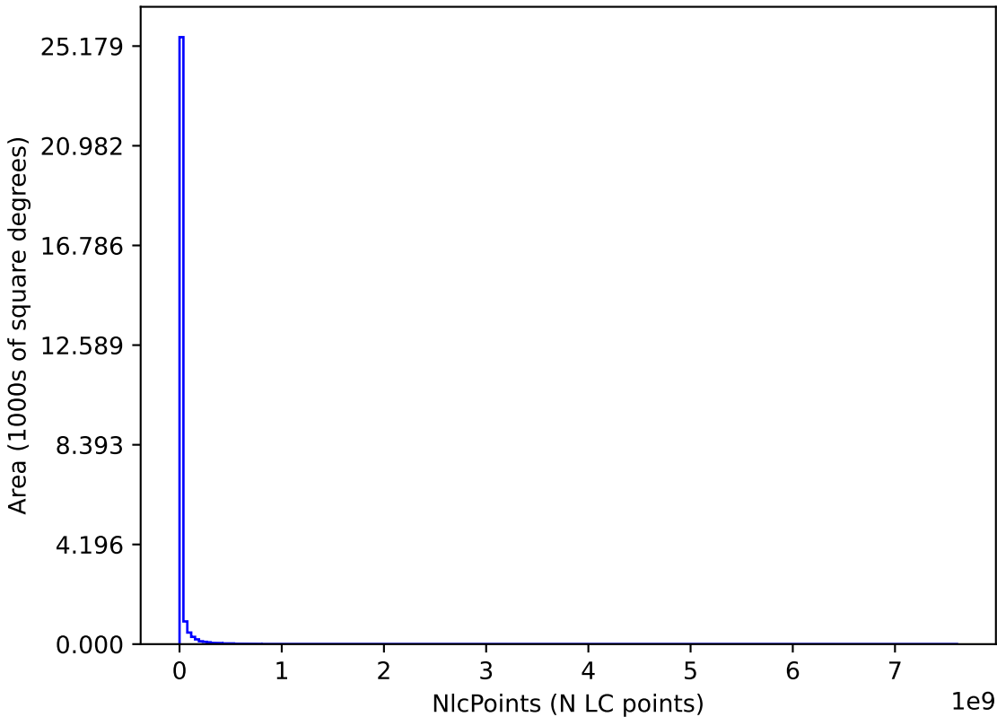
four_cycle_v3.6_10yrs : NlcPoints
