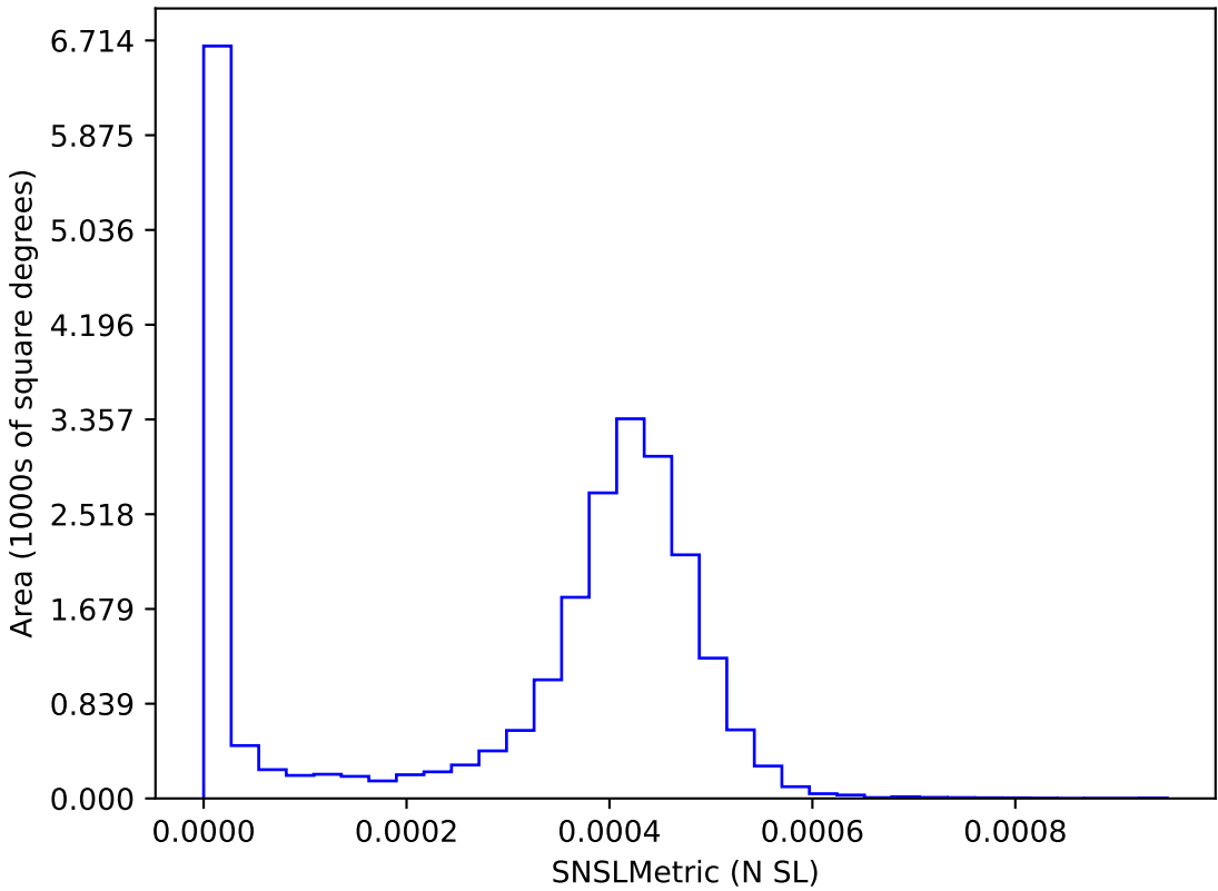
four_cycle_v3.6_10yrs : SNSLMetric
