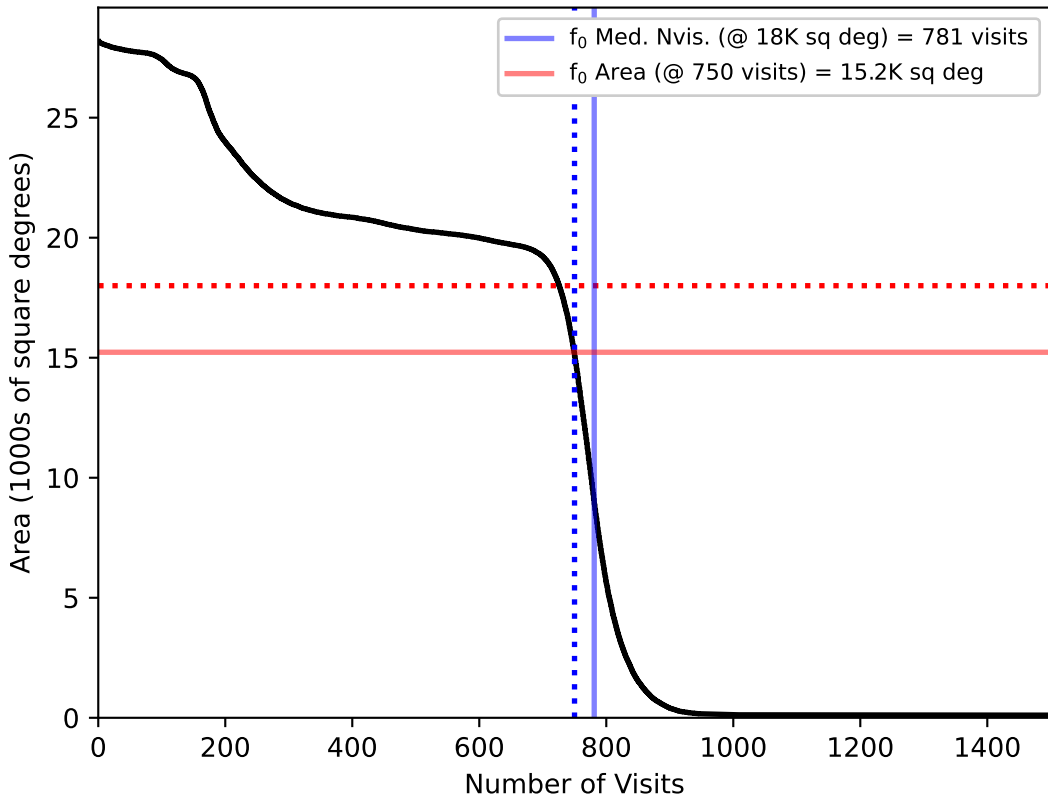
four_cycle_v4.0_10yrs : f0
