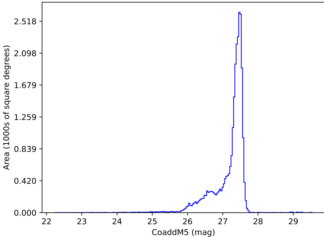
no_too_v3.6_10yrs : CoaddM5
