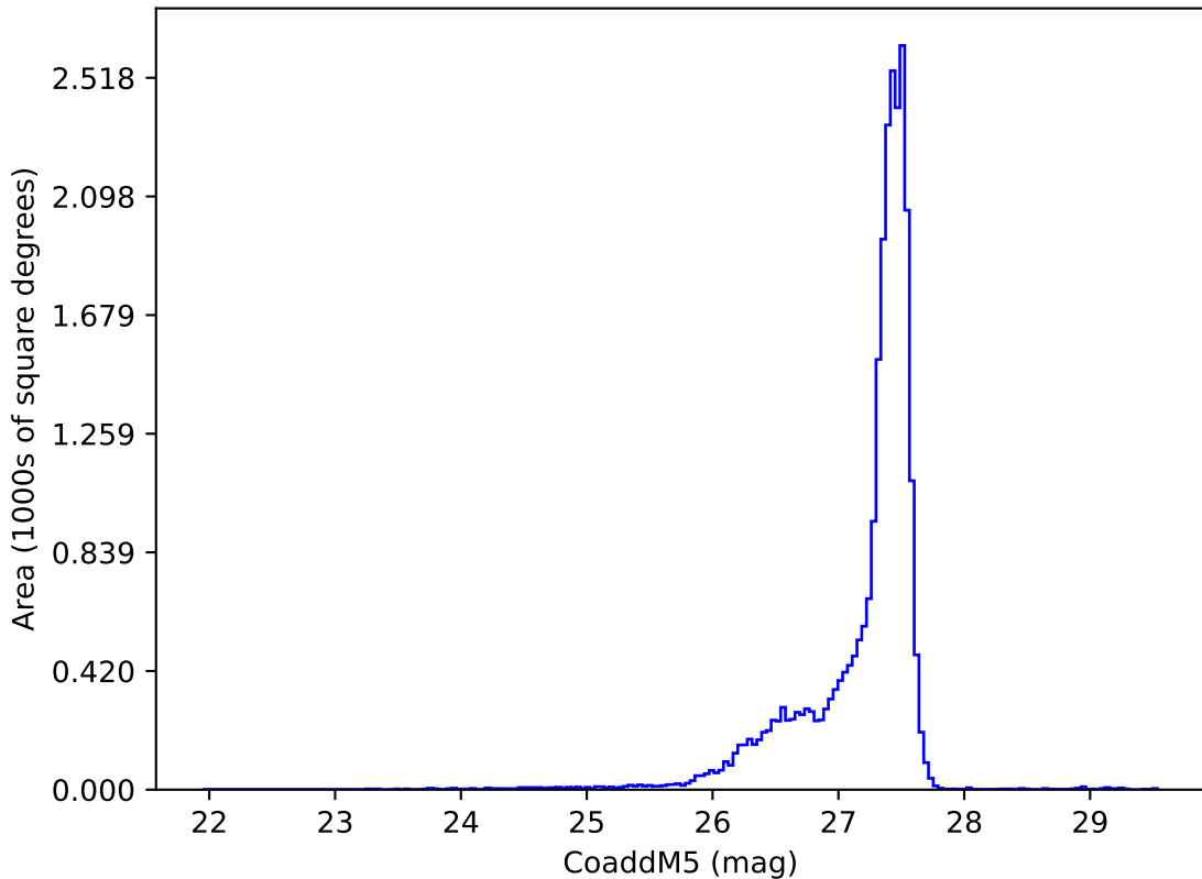
no_too_v4.0_10yrs : CoaddM5
