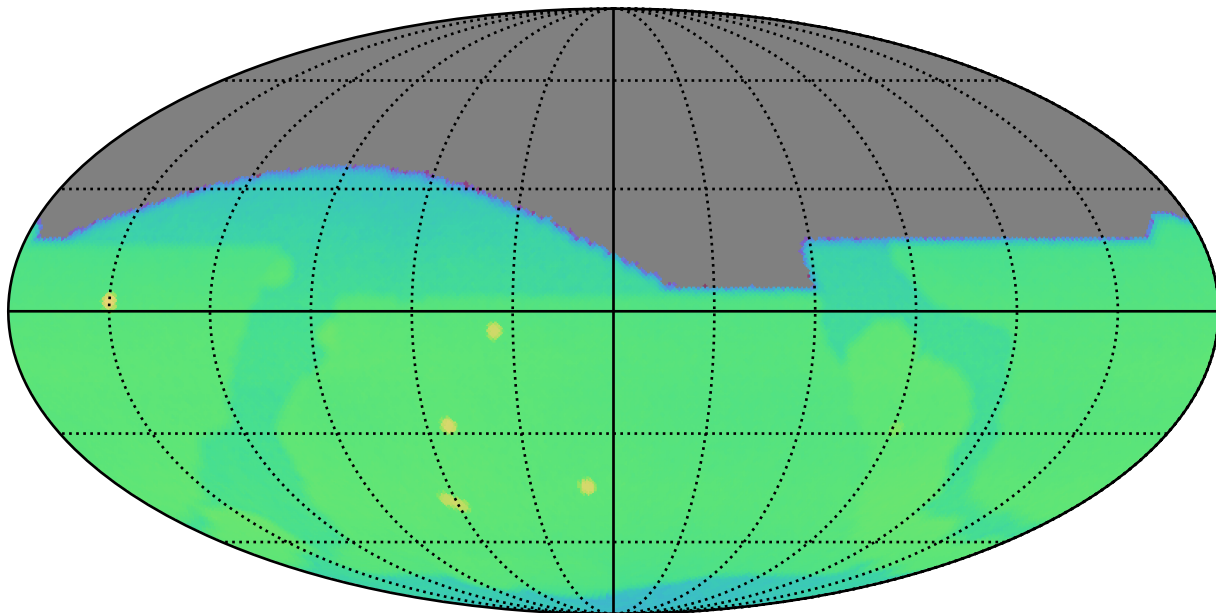
no_too_v4.0_10yrs : CoaddM5
