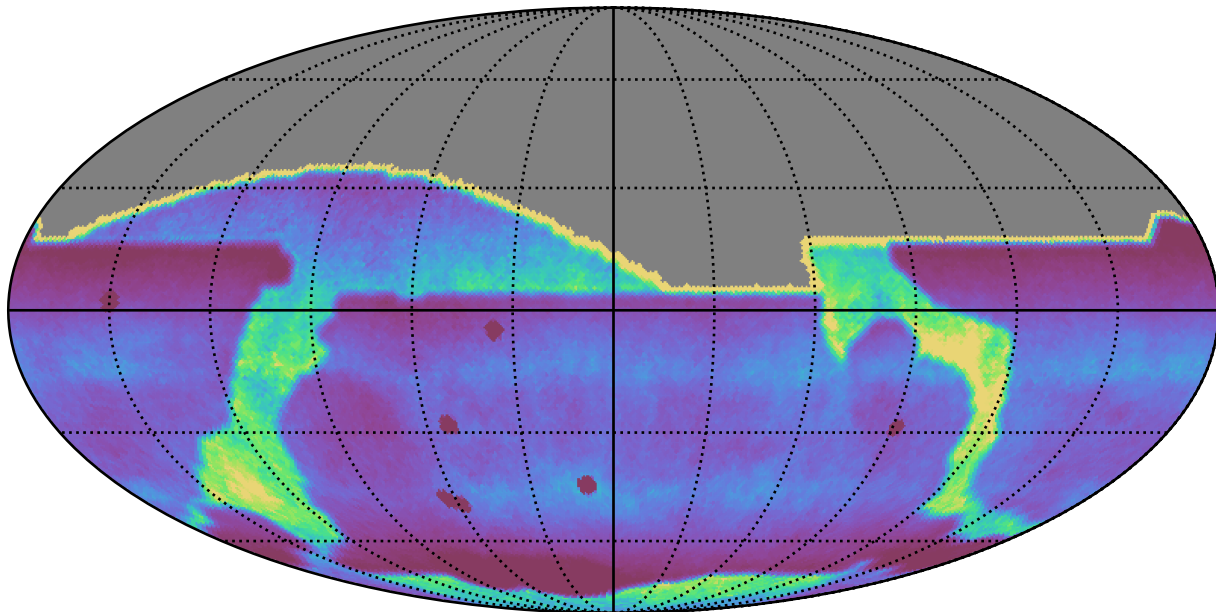
one_snap_v4.0_10yrs : DCRprecision
