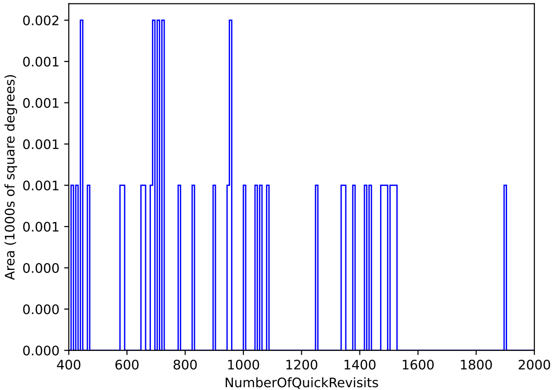
one_snap_v4.0_10yrs : NumberOfQuickRevisits
