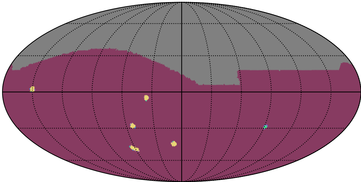
one_snap_v4.0_10yrs : NumberOfQuickRevisits
