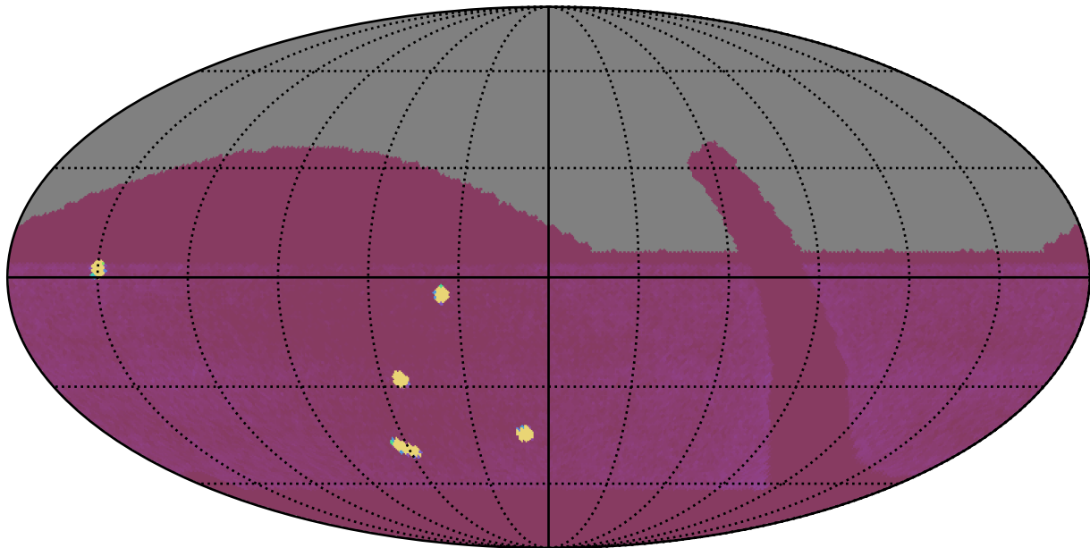
retro_baseline_v2.0_10yrs : NumberOfQuickRevisits
