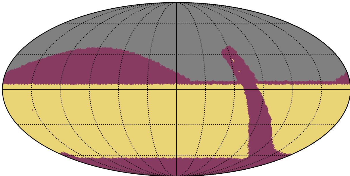
retro_baseline_v2.0_10yrs : RapidRevisits
