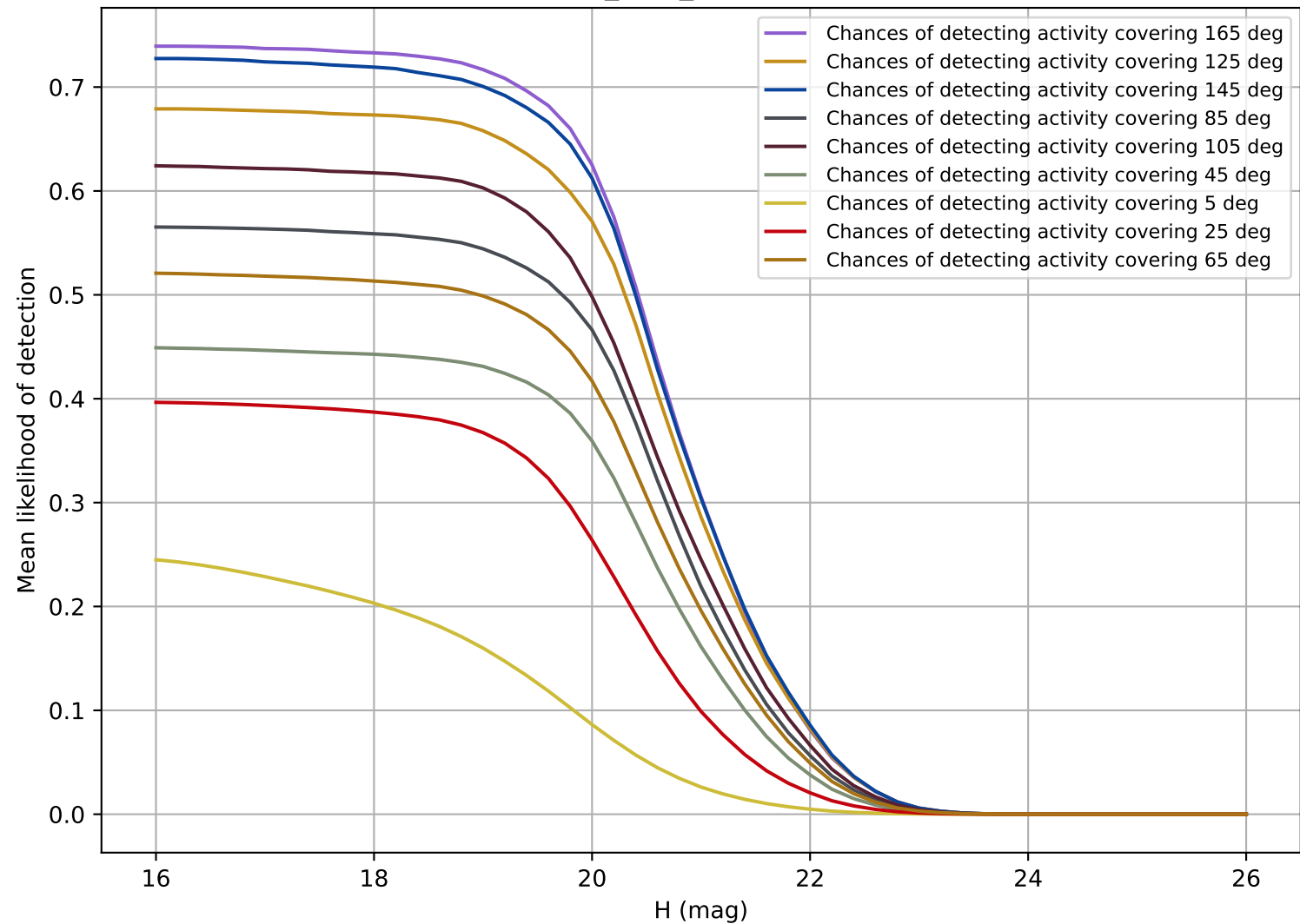
too_v3.5_10yrs MBA
