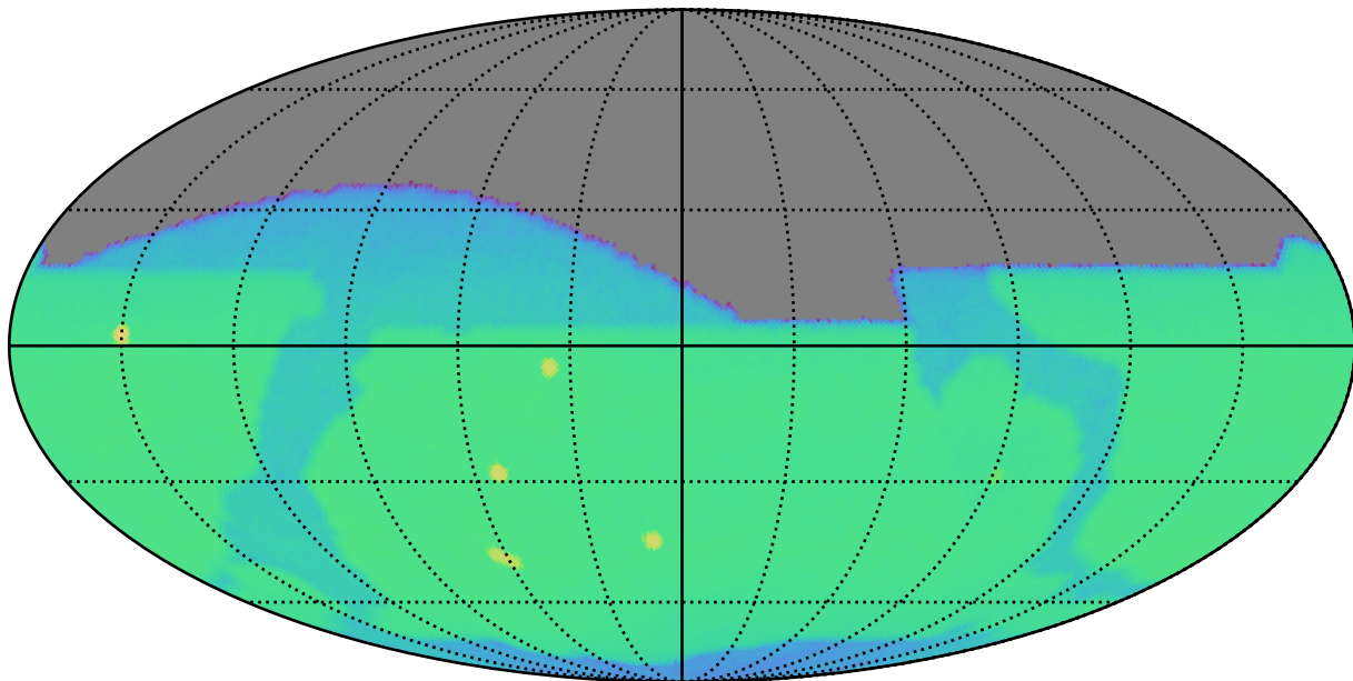
weather_cloudso0v3.5_10yrs i: CoaddM5
