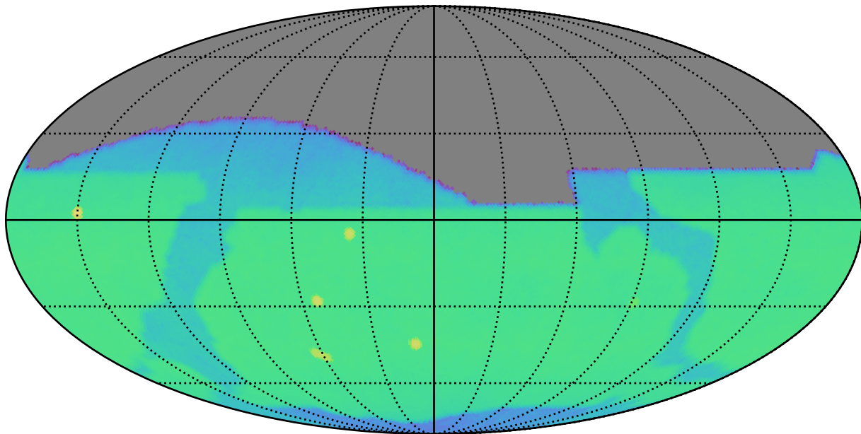
weather_cloudso10v3.5_10yrs i: CoaddM5
