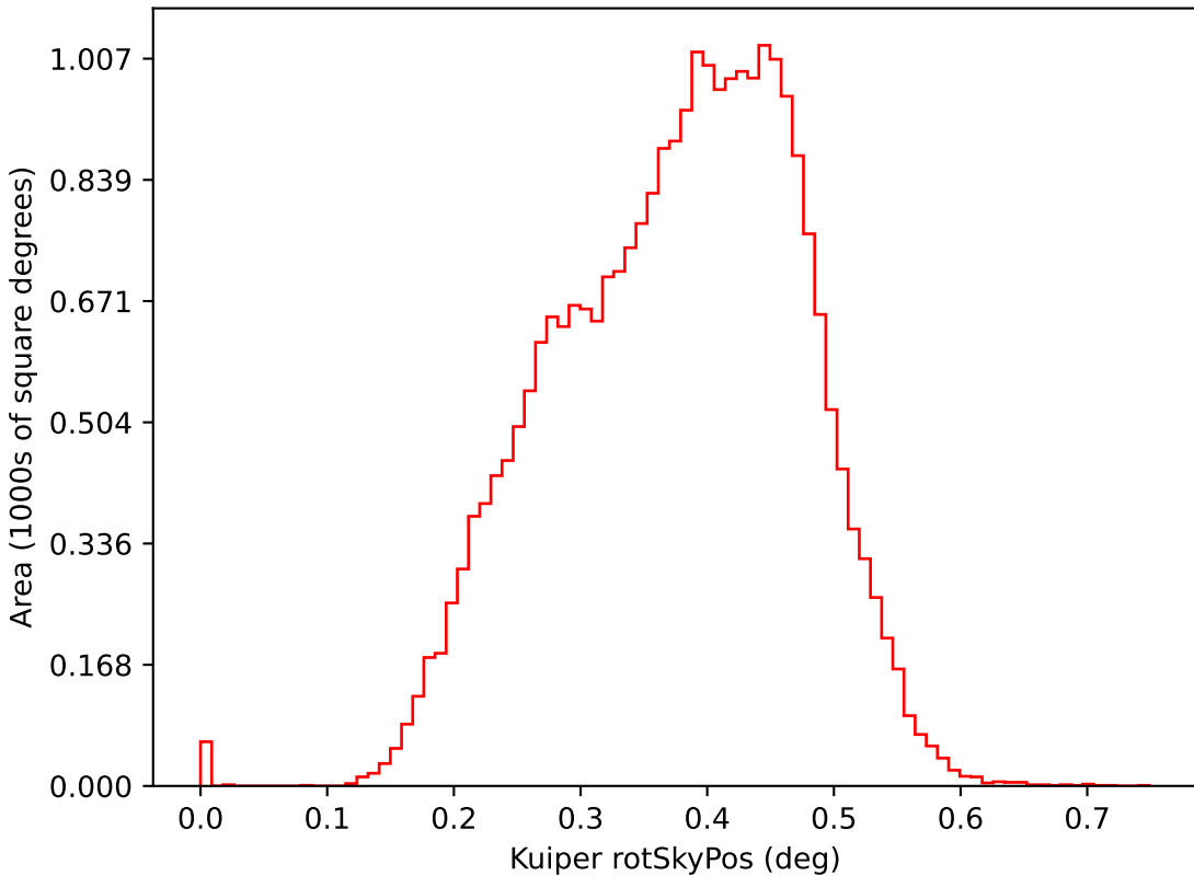
weather_cloudso12v3.5_10yrs i: Kuiper rotSkyPos
