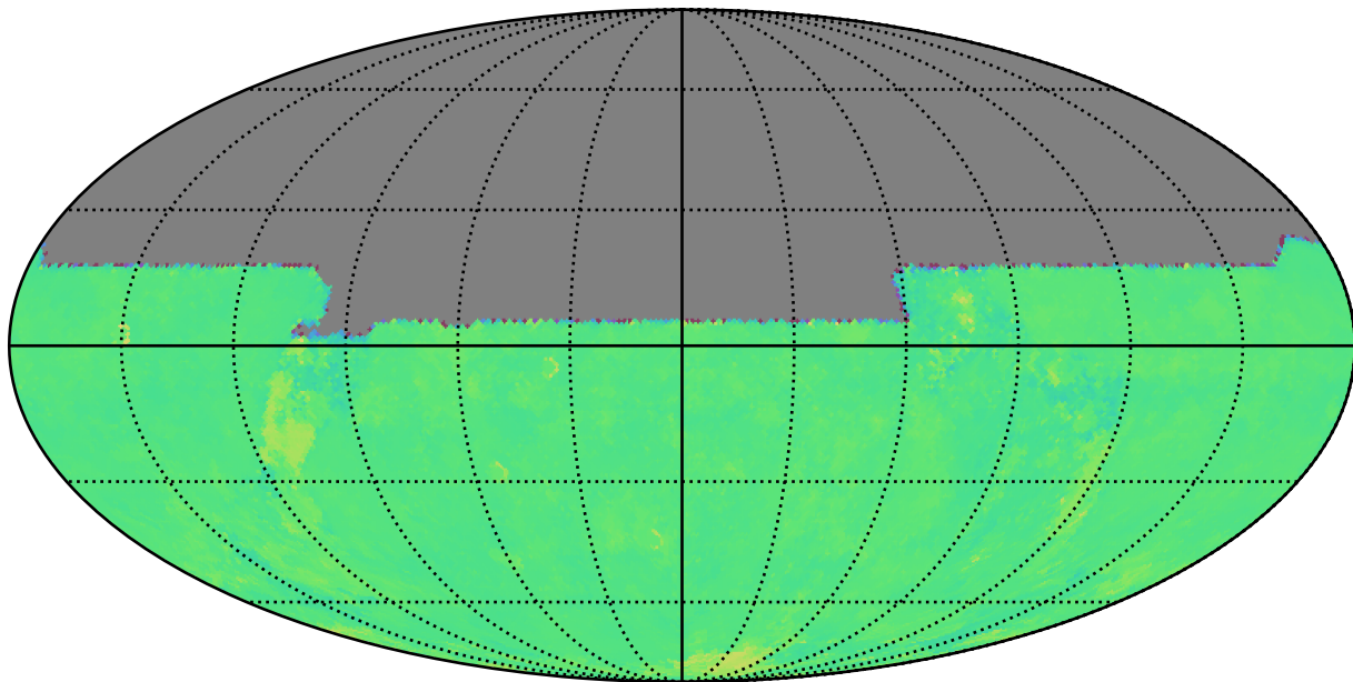
weather_cloudso12v3.5_10yrs u: Kuiper rotTelPos
