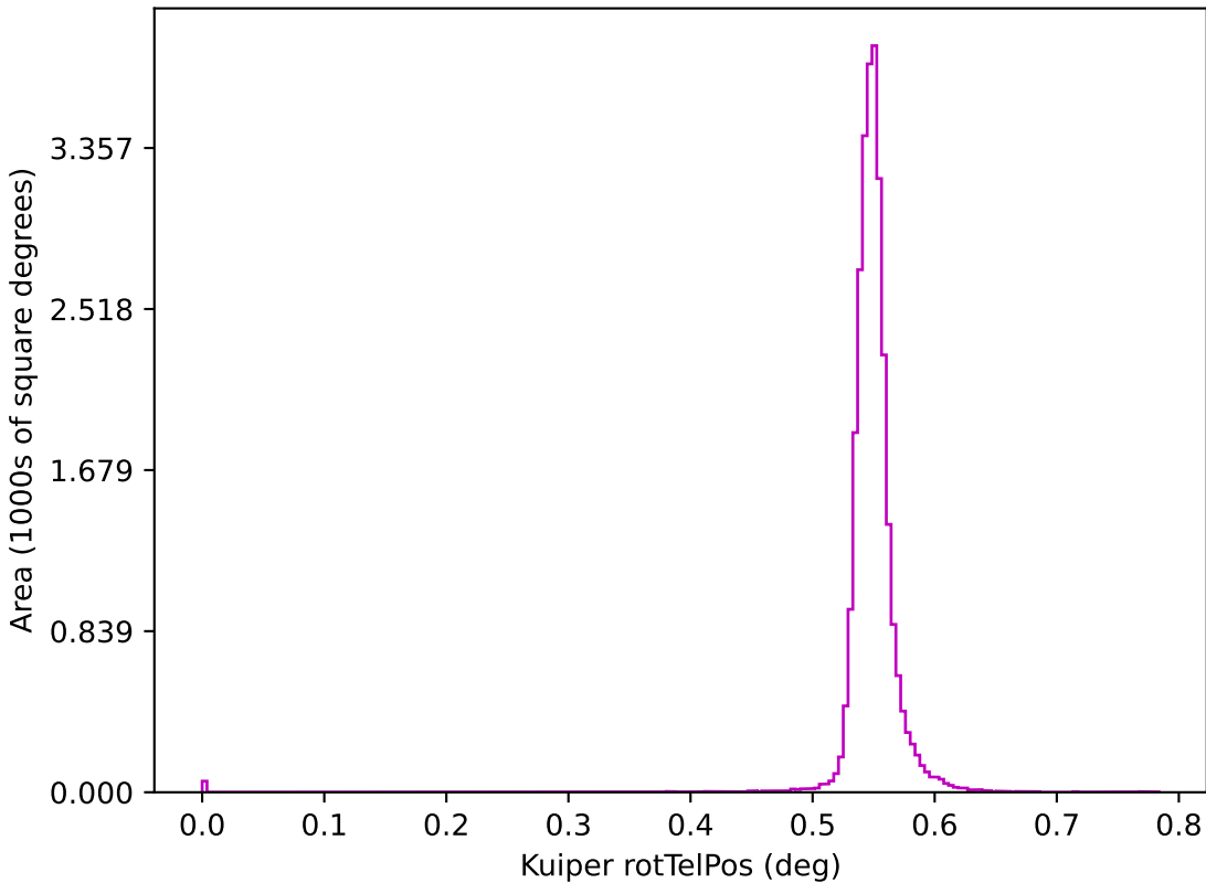
weather_cloudso12v3.5_10yrs z: Kuiper rotTelPos
