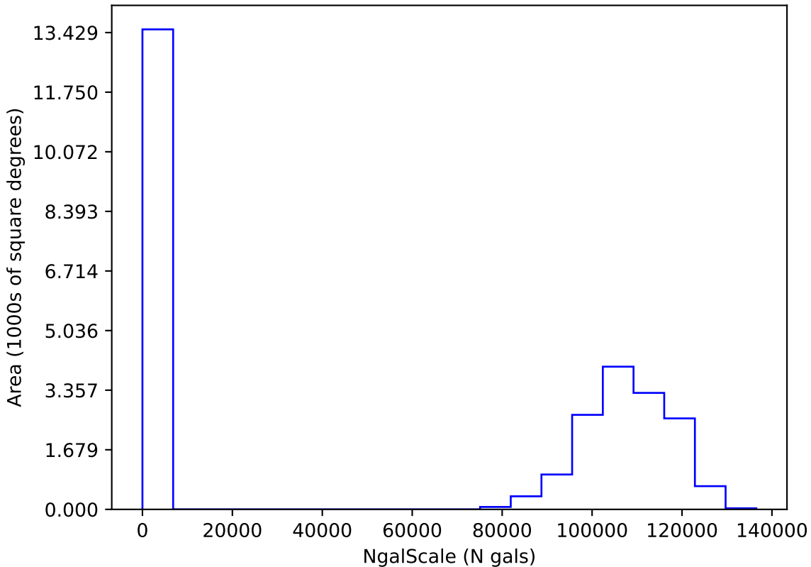
weather_cloudso12v3.5_10yrs i: NgalScale
