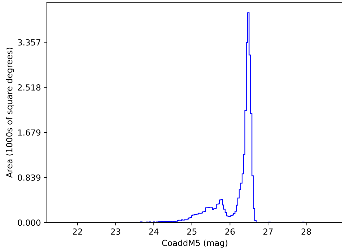
weather_cloudso14v3.5_10yrs i: CoaddM5
