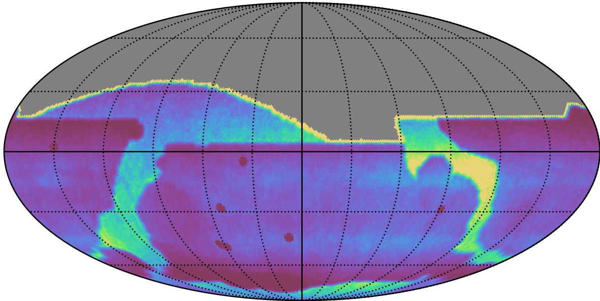
weather_cloudso14v3.5_10yrs : DCRprecision
