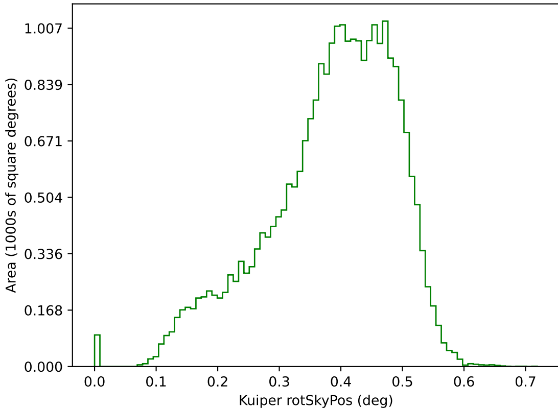
weather_cloudso14v3.5_10yrs g: Kuiper rotSkyPos
