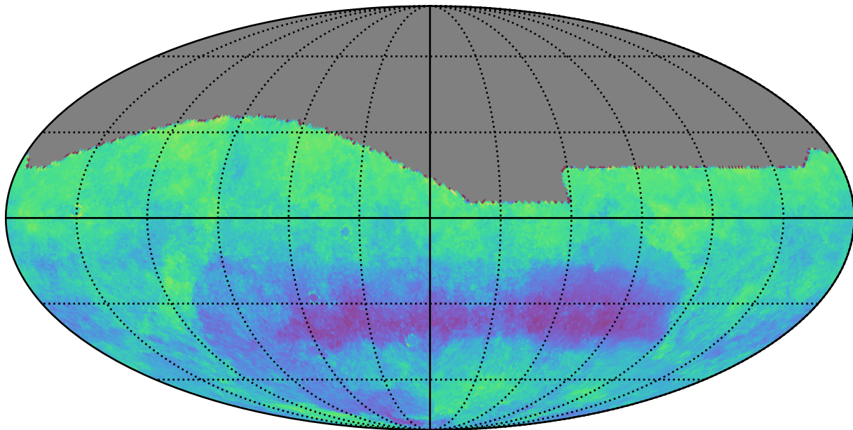
weather_cloudso14v3.5_10yrs g: Kuiper rotSkyPos
