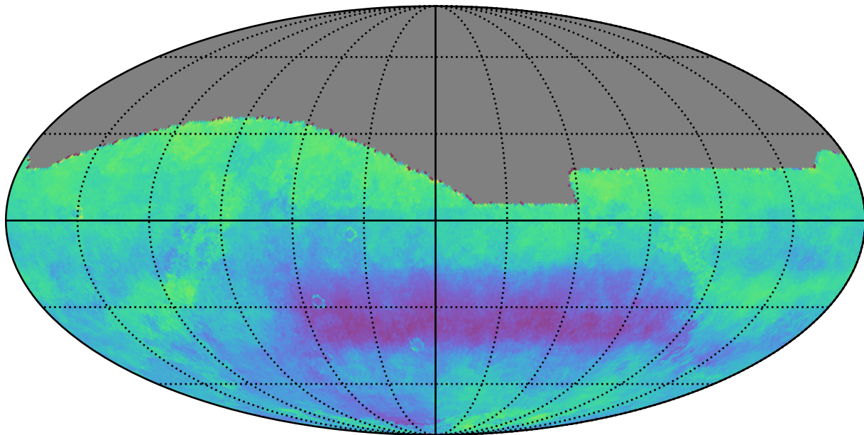
weather_cloudso14v3.5_10yrs r: Kuiper rotSkyPos
