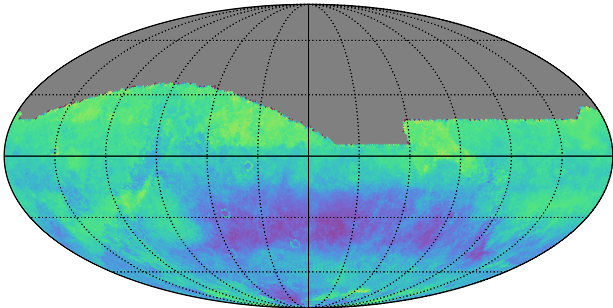
weather_cloudso14v3.5_10yrs z: Kuiper rotSkyPos
