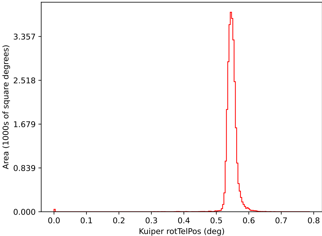
weather_cloudso14v3.5_10yrs i: Kuiper rotTelPos
