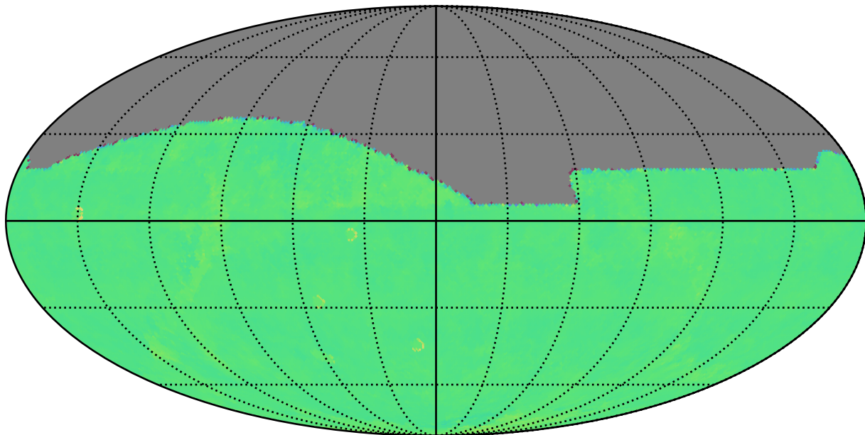
weather_cloudso14v3.5_10yrs r: Kuiper rotTelPos
