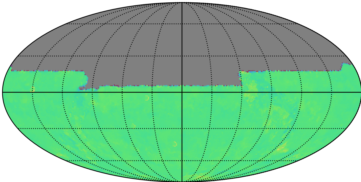
weather_cloudso14v3.5_10yrs u: Kuiper rotTelPos
