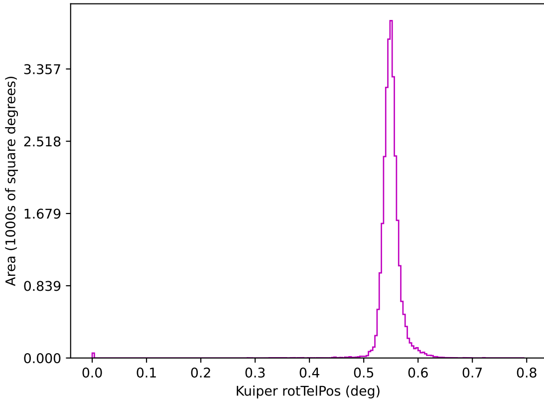
weather_cloudso14v3.5_10yrs z: Kuiper rotTelPos
