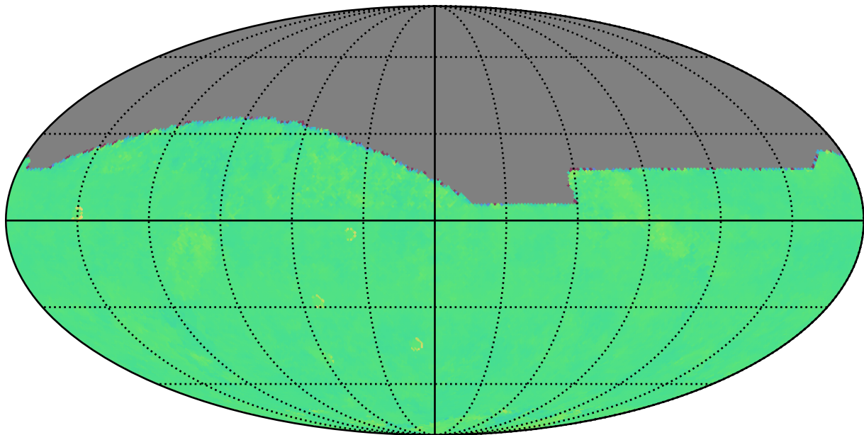
weather_cloudso14v3.5_10yrs z: Kuiper rotTelPos
