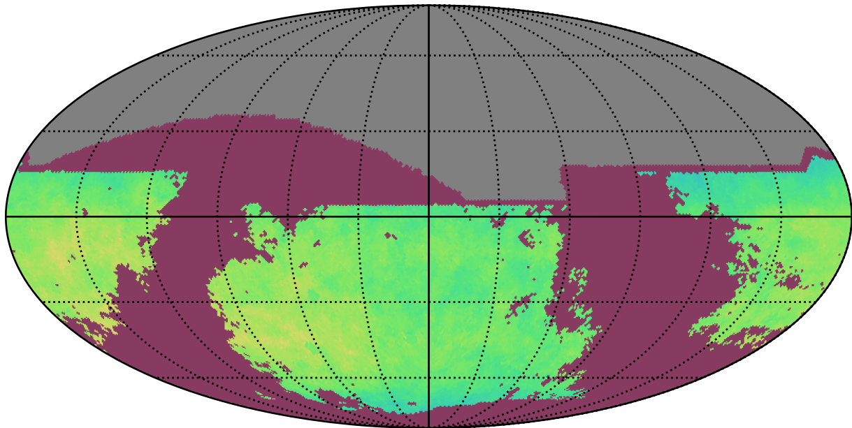
weather_cloudso14v3.5_10yrs i: NgalScale
