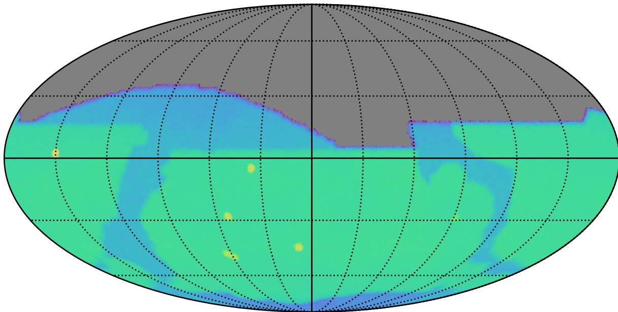
weather_cloudso14v3.5_10yrs i: SurfaceBrightLimit
