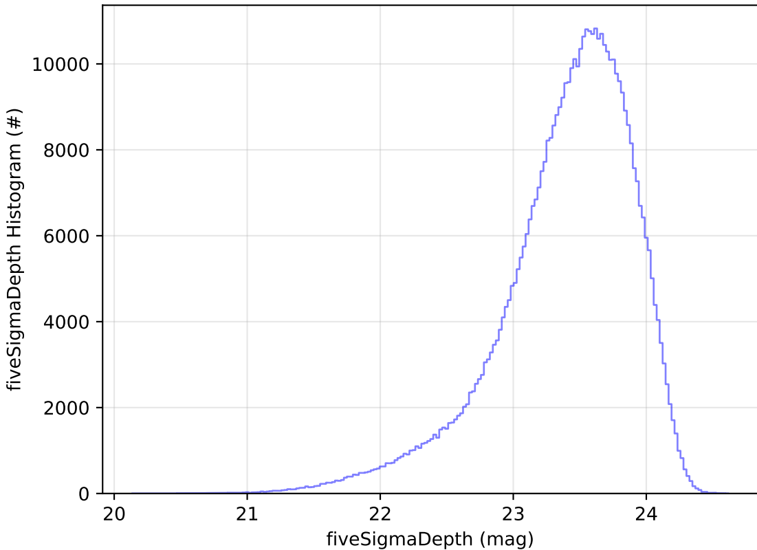
weather_cloudso14v3.5_10yrs i: fiveSigmaDepth Histogram
