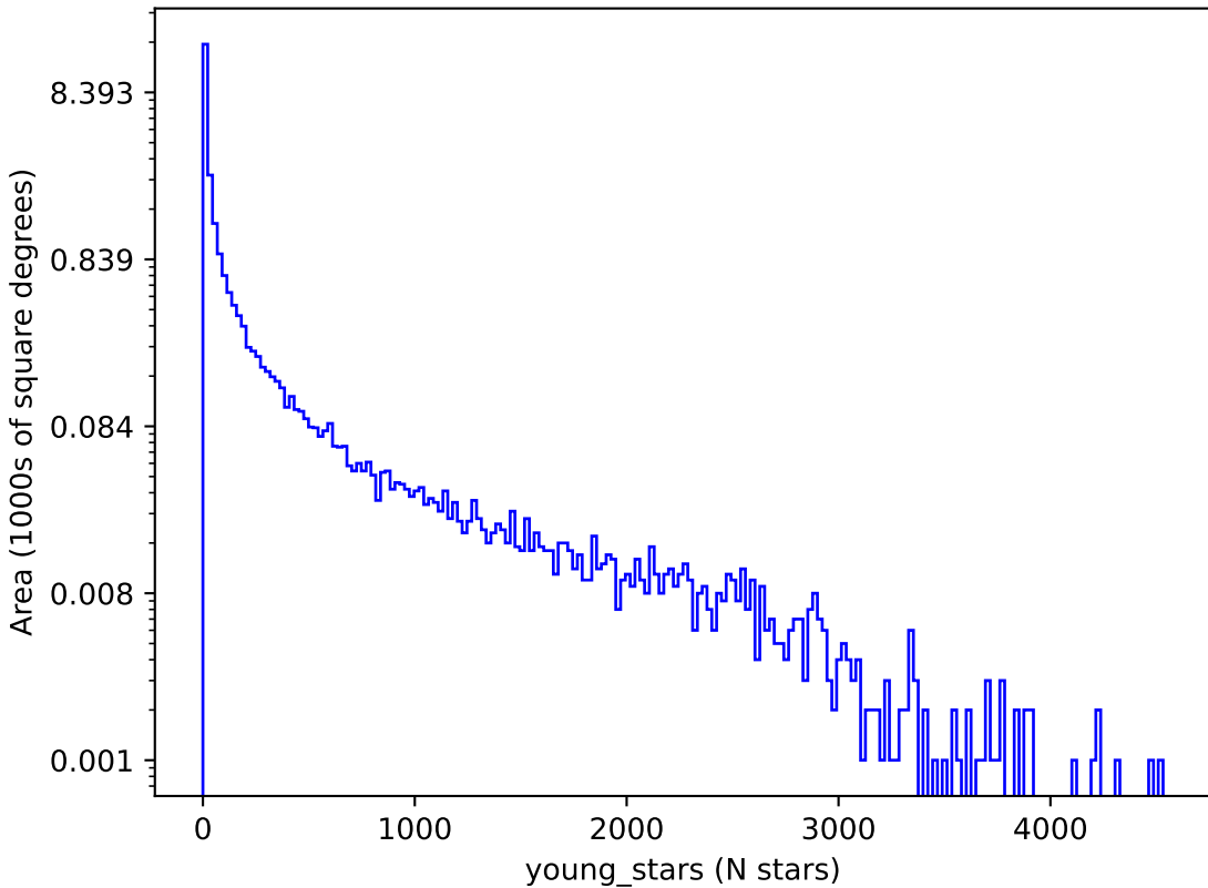
weather_cloudso14v3.5_10yrs : young_stars
