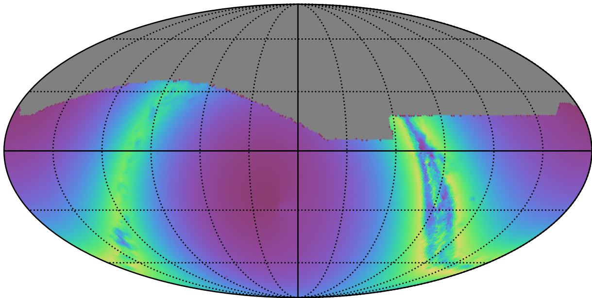
weather_cloudso14v3.5_10yrs : young_stars
