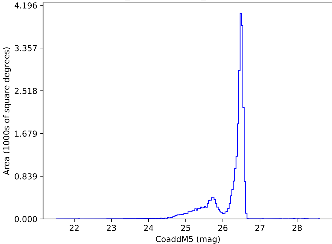
weather_cloudso16v3.5_10yrs i: CoaddM5
