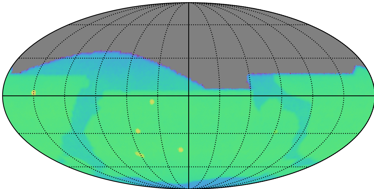
weather_cloudso16v3.5_10yrs i: CoaddM5
