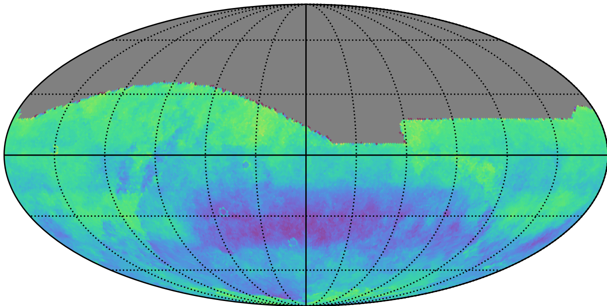
weather_cloudso16v3.5_10yrs i: Kuiper rotSkyPos
