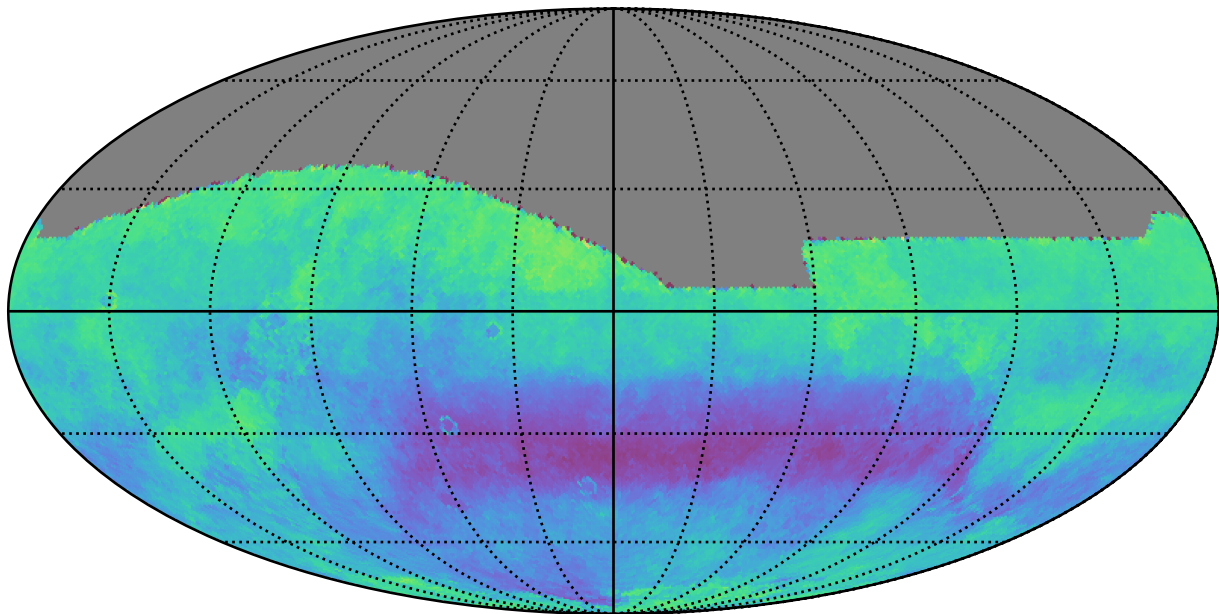
weather_cloudso16v3.5_10yrs r: Kuiper rotSkyPos
