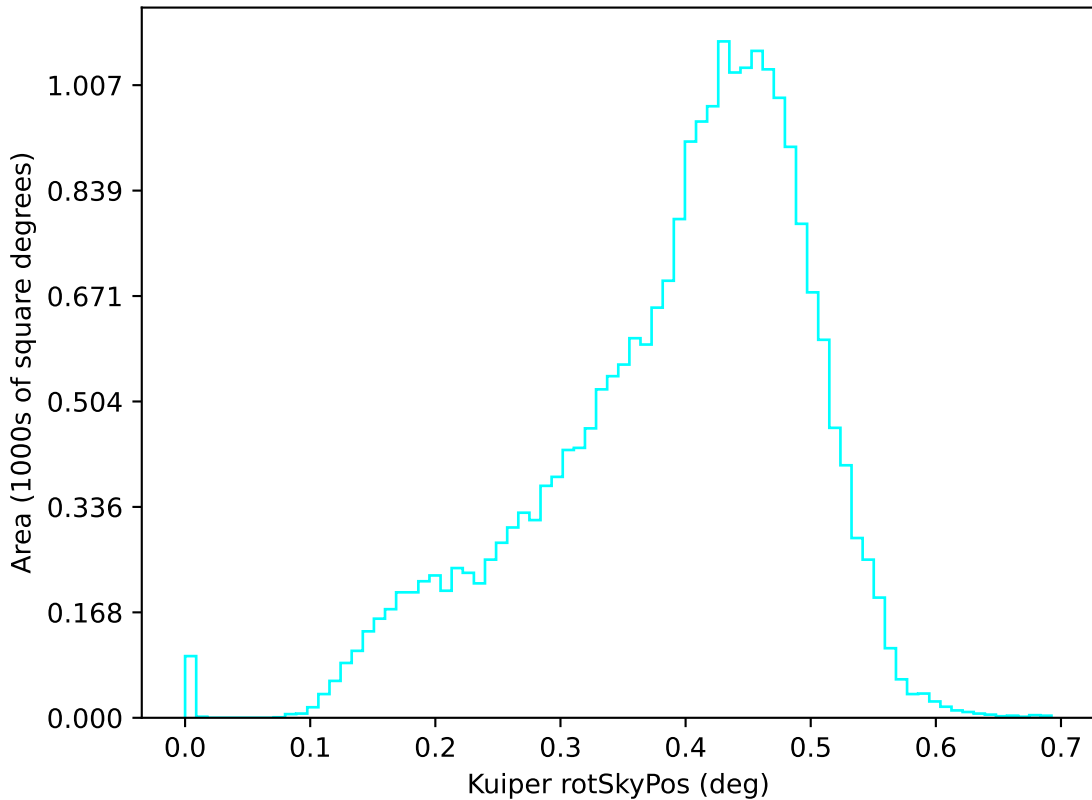
weather_cloudso16v3.5_10yrs u: Kuiper rotSkyPos
