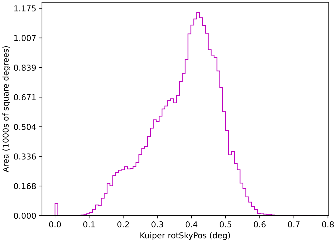
weather_cloudso16v3.5_10yrs z: Kuiper rotSkyPos
