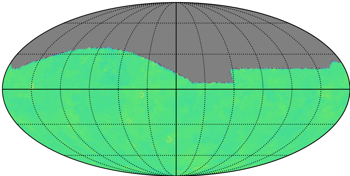
weather_cloudso16v3.5_10yrs g: Kuiper rotTelPos
