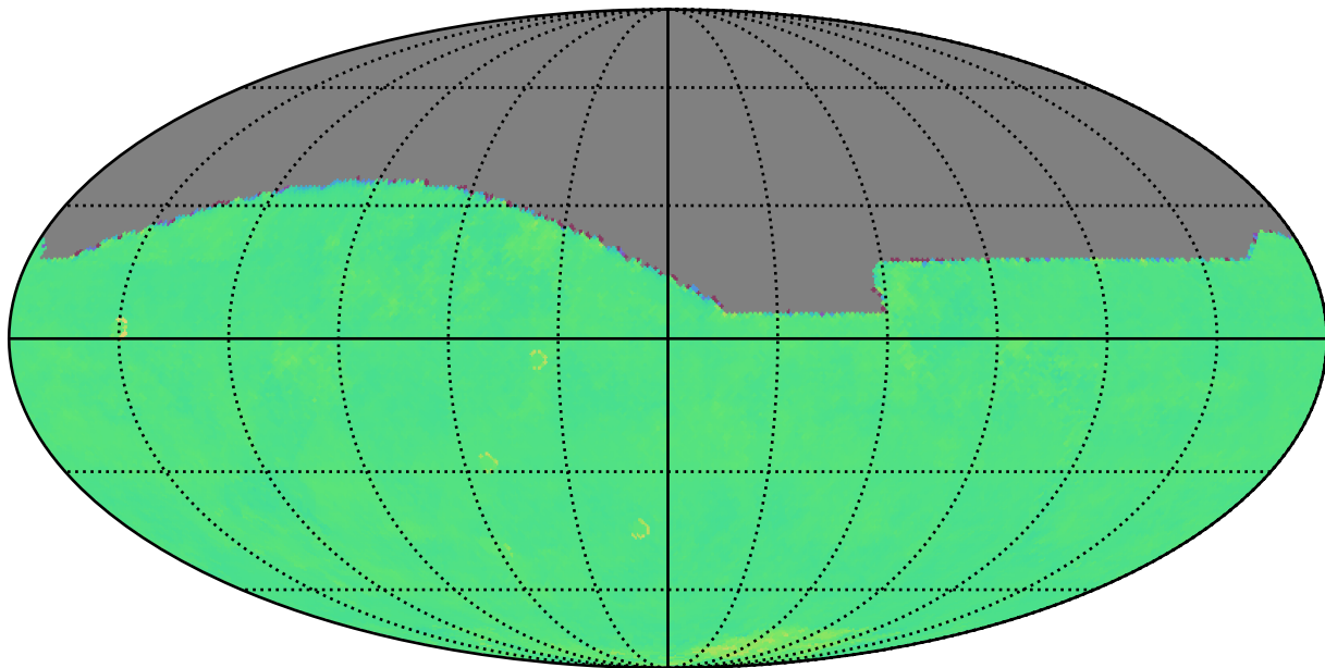
weather_cloudso16v3.5_10yrs i: Kuiper rotTelPos
