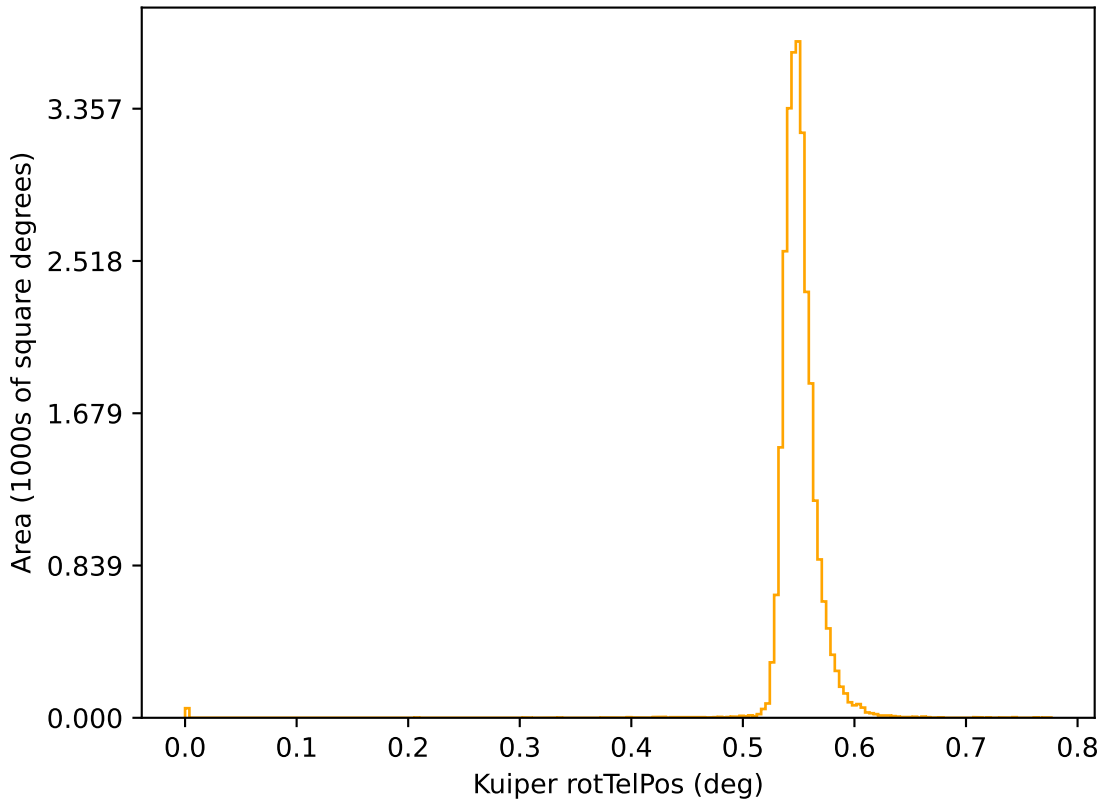
weather_cloudso16v3.5_10yrs r: Kuiper rotTelPos
