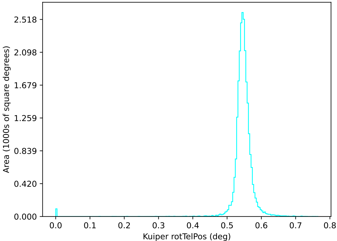
weather_cloudso16v3.5_10yrs u: Kuiper rotTelPos
